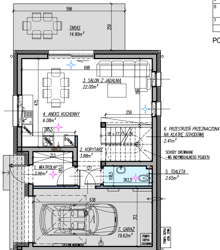
RZUT PARTERU
