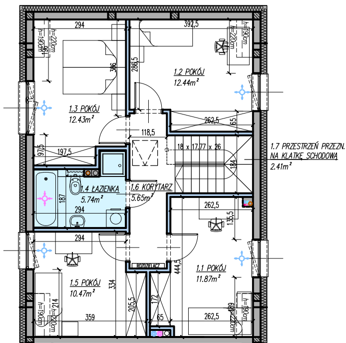
RZUT PODDASZA
